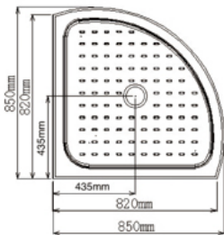
RC820/870
